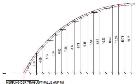
Abb. 3 Beispielhafte Schnitte einer Traglufthalle für Tennisplätze. Darstellung: DUOL 2026
